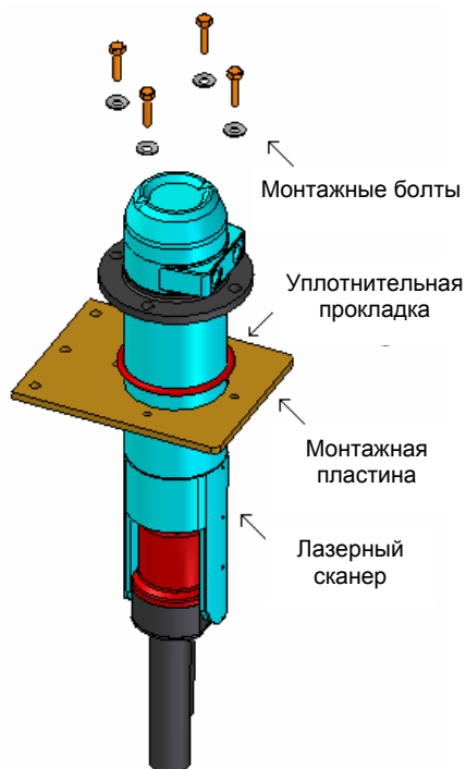
Рисунок 20 – Монтажный набор LM3D.
