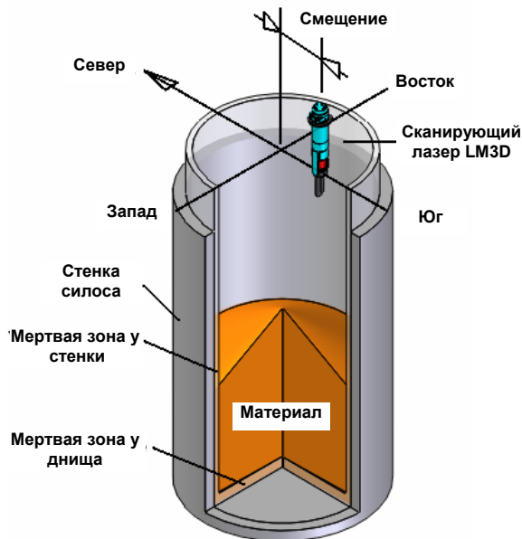
Рисунок 8 - Типовая схема монтажа.
