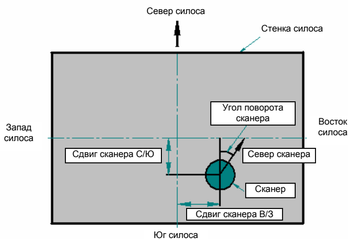
Рисунок 19 – Сканер установлен на прямоугольном силосе.
