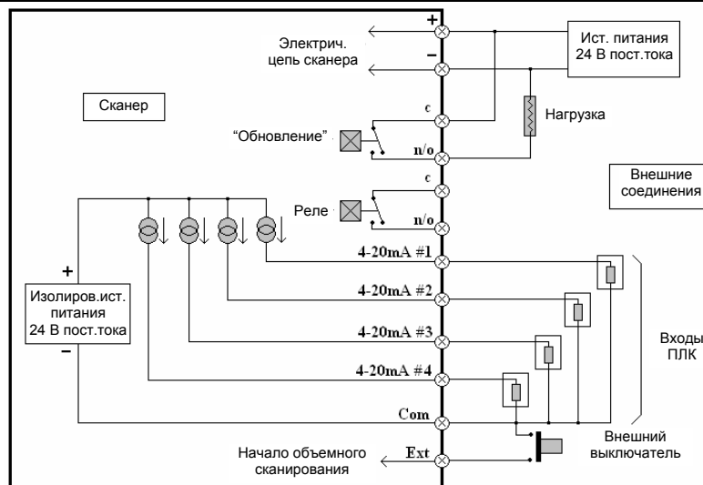
Рисунок 15 – Схема электрических соединений.
