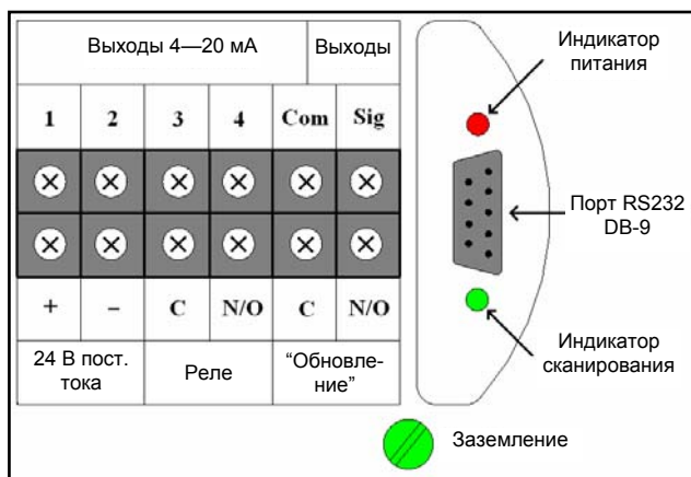
Рисунок 14 – Клеммный отсек.
