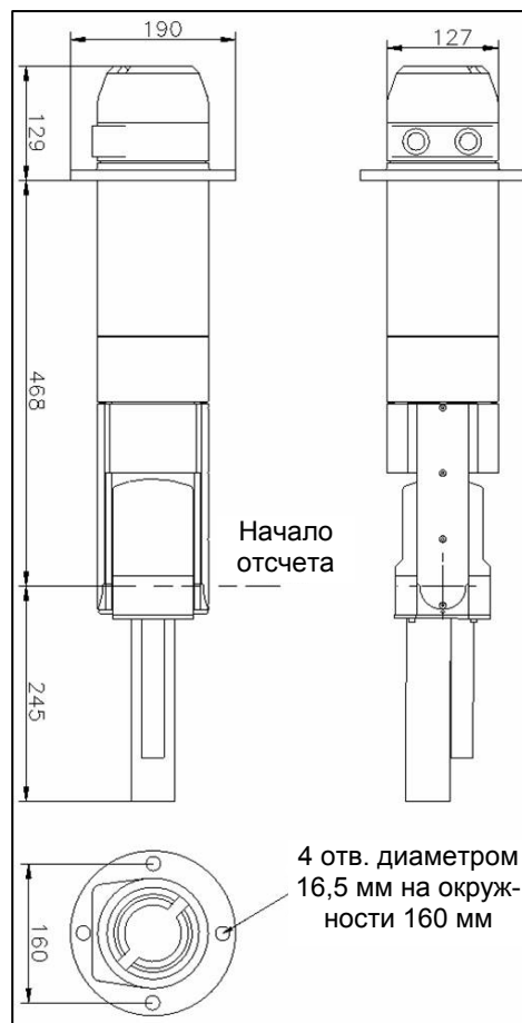
Рисунок 7 – Габаритные размеры.
