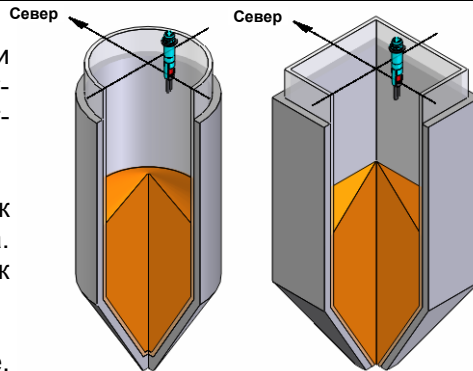
Рисунок 9 - Установка сканирующего лазера LM3D.
