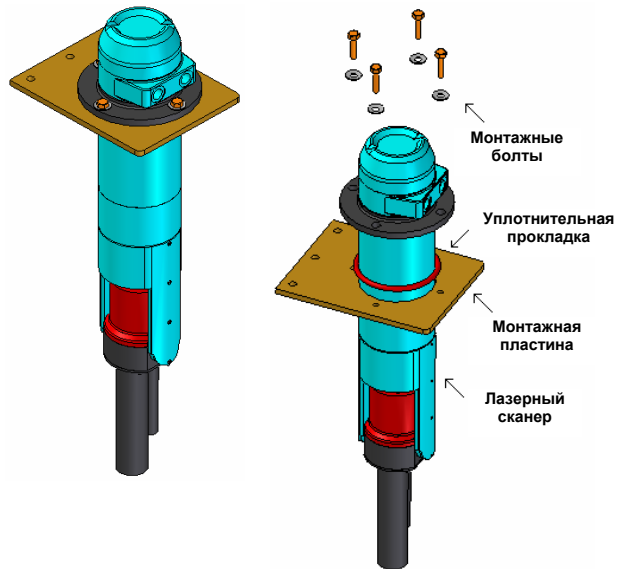
Рисунок 11 – Регулируемый монтажный кронштейн.
